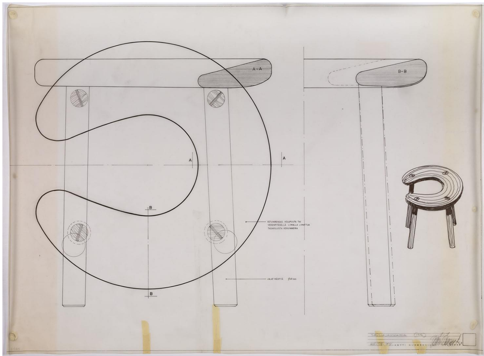
Antti Nurmesniemi, Saunajakkara Hotelli Palacen saunaosastolle, tekninen piirros 1952.
